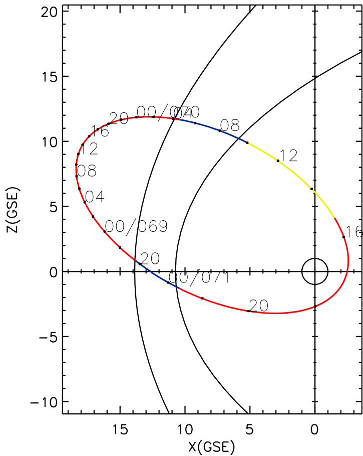
CLUSTER 2 orbit 2023 068 (03/09) 19:01 UT to 2023 071 (03/12) 01:16 UT
