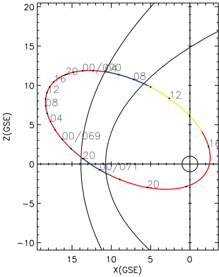
CLUSTER 2 orbit 2023 068 (03/09) 18:51 UT to 2023 071 (03/12) 01:06 UT
