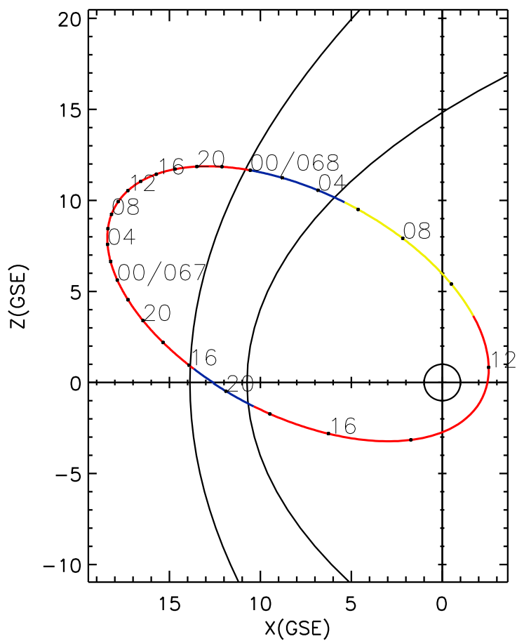
CLUSTER 2 orbit 2023 066 (03/07) 14:26 UT to 2023 068 (03/09) 20:41 UT
