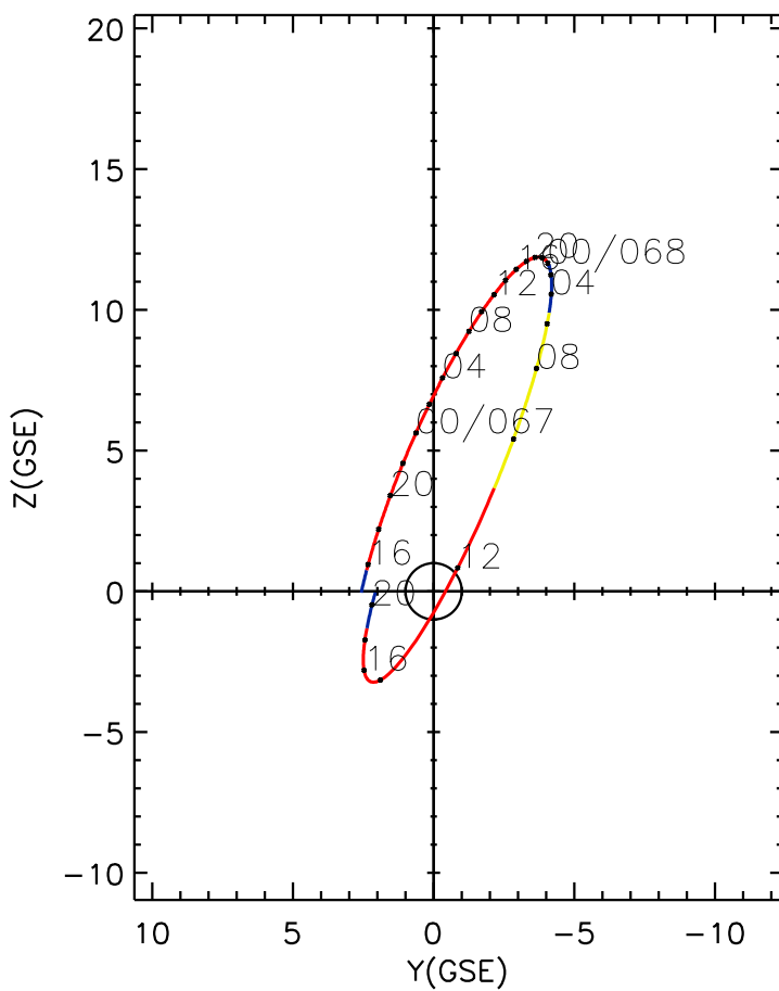
CLUSTER 2 orbit 2023 066 (03/07) 14:26 UT to 2023 068 (03/09) 20:41 UT
