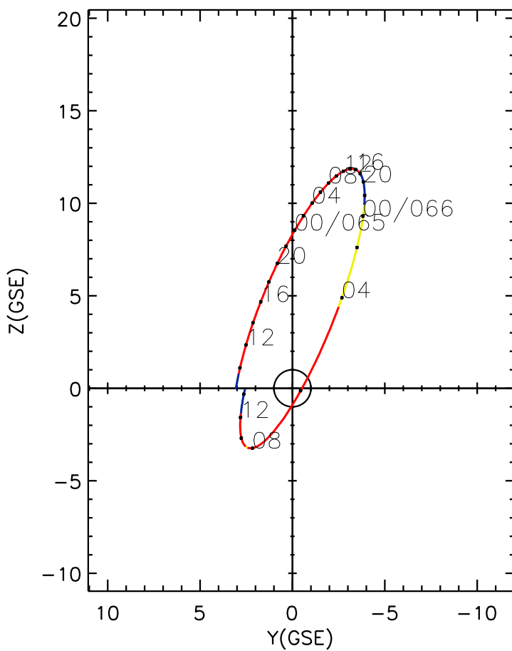
CLUSTER 2 orbit 2023 064 (03/05) 08:11 UT to 2023 066 (03/07) 14:26 UT
