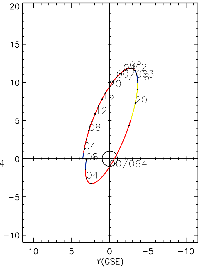
CLUSTER 2 orbit 2023 062 (03/03) 01:56 UT to 2023 064 (03/05) 08:11 UT
