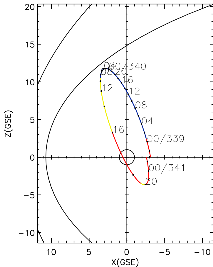
CLUSTER 2 orbit 2022 338 (12/04) 20:41 UT to 2022 341 (12/07) 02:56 UT
