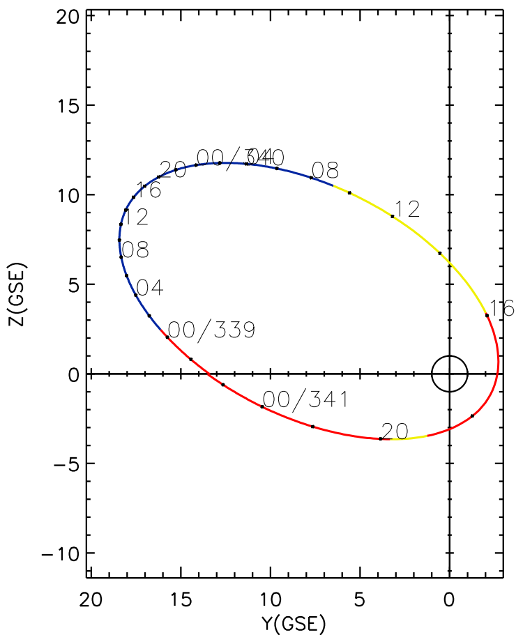
CLUSTER 2 orbit 2022 338 (12/04) 20:41 UT to 2022 341 (12/07) 02:56 UT
