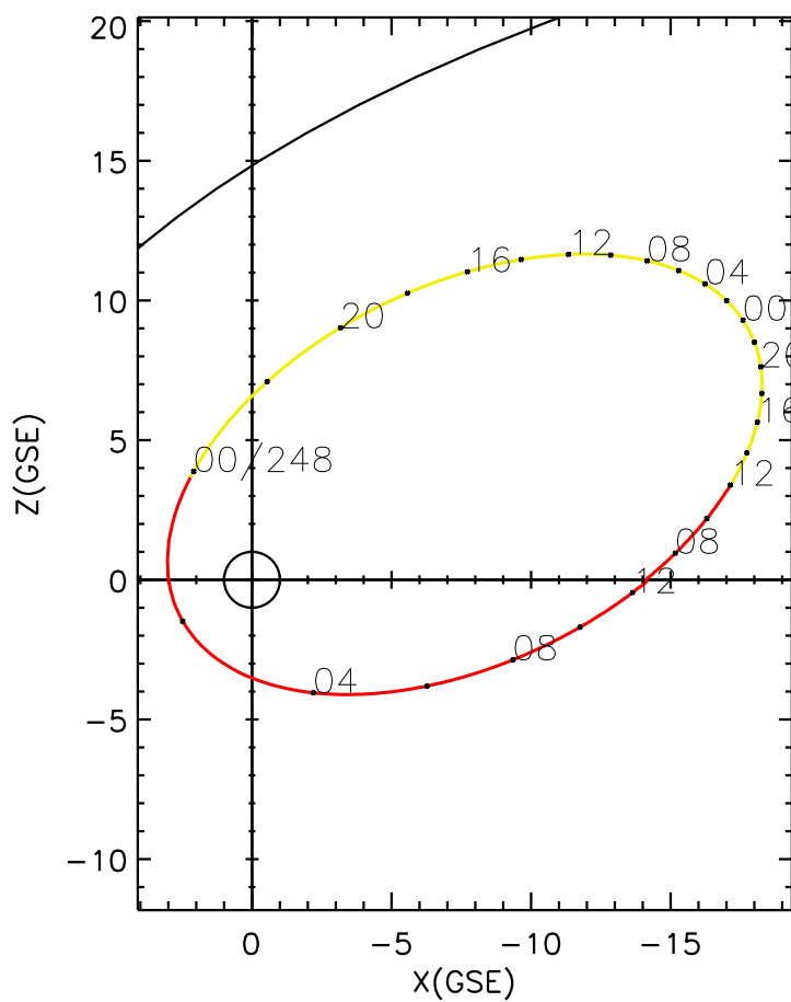
CLUSTER 2 orbit 2022 246 (09/03) 06:26 UT to 2022 248 (09/05) 12:41 UT
