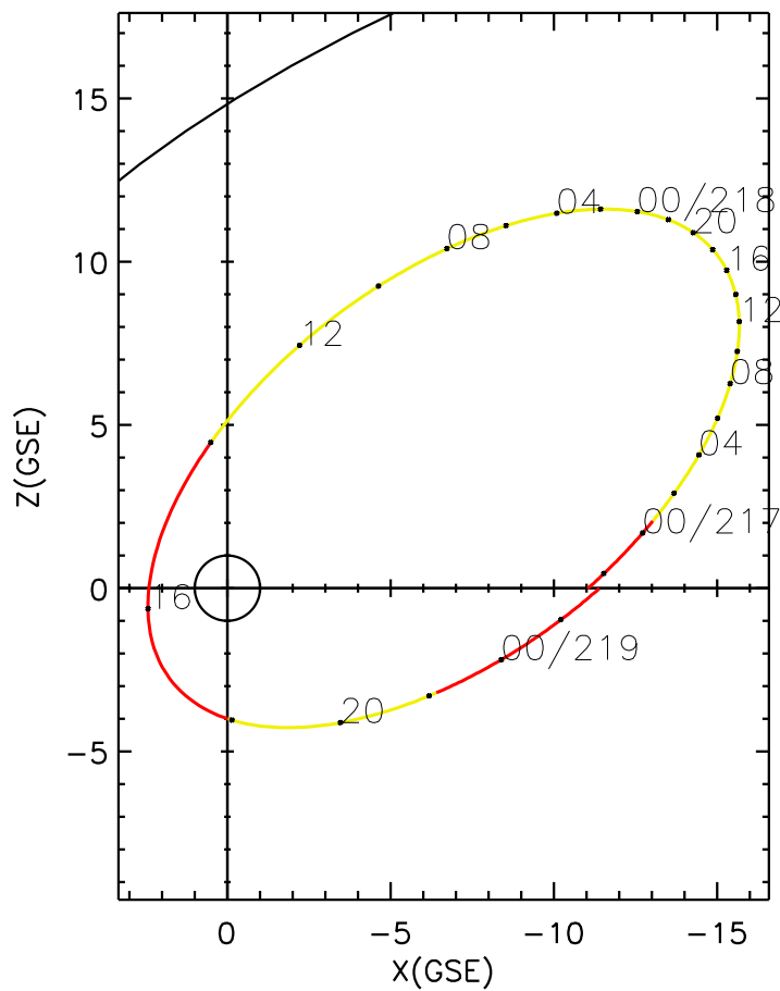
CLUSTER 2 orbit 2022 216 (08/04) 21:16 UT to 2022 219 (08/07) 03:31 UT
