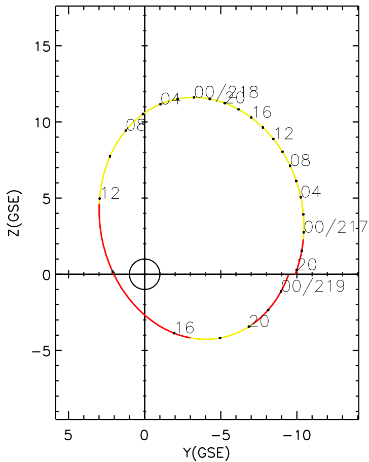
CLUSTER 2 orbit 2022 216 (08/04) 19:31 UT to 2022 219 (08/07) 01:46 UT
