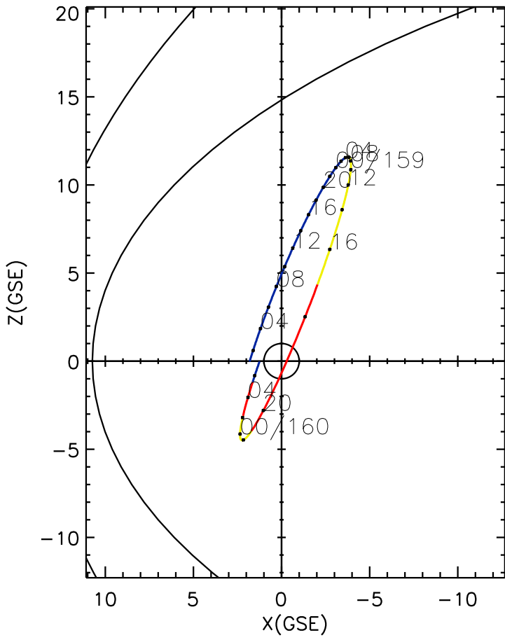
CLUSTER 2 orbit 2022 158 (06/07) 01:01 UT to 2022 160 (06/09) 07:16 UT
