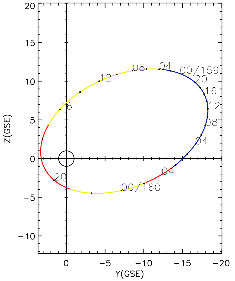
CLUSTER 2 orbit 2022 158 (06/07) 01:01 UT to 2022 160 (06/09) 07:16 UT
