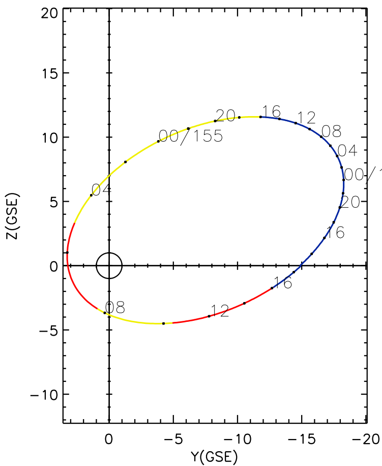
CLUSTER 2 orbit 2022 153 (06/02) 12:31 UT to 2022 155 (06/04) 18:46 UT
