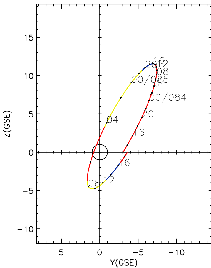
CLUSTER 2 orbit 2022 083 (03/24) 12:31 UT to 2022 085 (03/26) 18:46 UT
