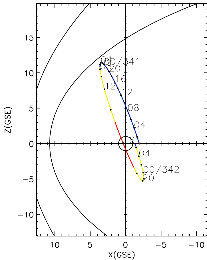
CLUSTER 2 orbit 2021 340 (12/06) 00:31 UT to 2021 342 (12/08) 06:46 UT
