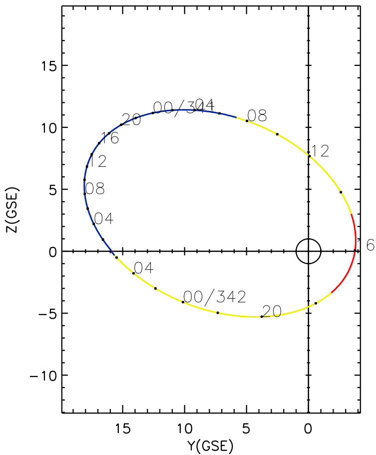
CLUSTER 2 orbit 2021 340 (12/06) 00:31 UT to 2021 342 (12/08) 06:46 UT
