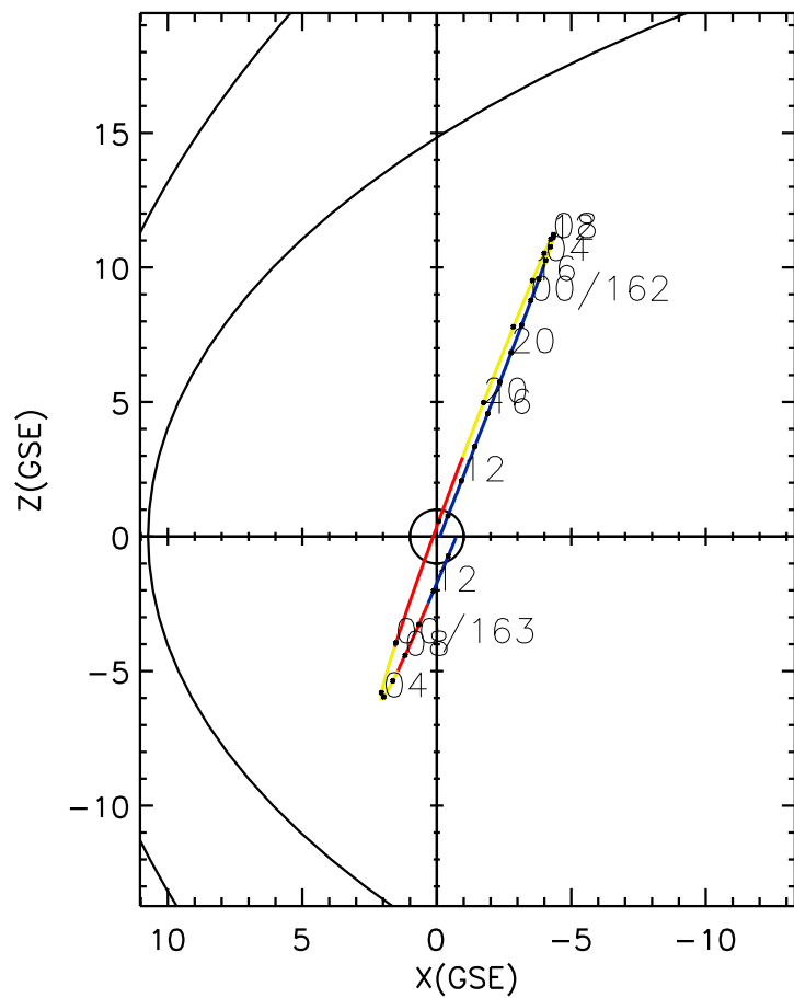
CLUSTER 2 orbit 2021 161 (06/10) 08:46 UT to 2021 163 (06/12) 15:01 UT
