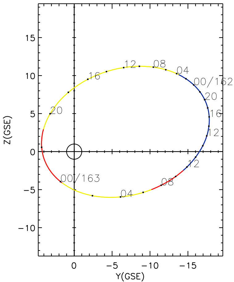
CLUSTER 2 orbit 2021 161 (06/10) 08:46 UT to 2021 163 (06/12) 15:01 UT
