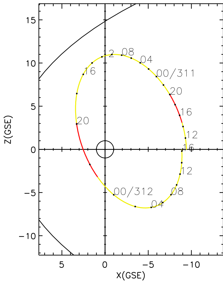
CLUSTER 2 orbit 2020 310 (11/05) 10:01 UT to 2020 312 (11/07) 16:16 UT
