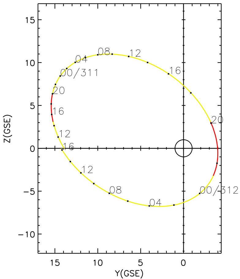
CLUSTER 2 orbit 2020 310 (11/05) 10:01 UT to 2020 312 (11/07) 16:16 UT
