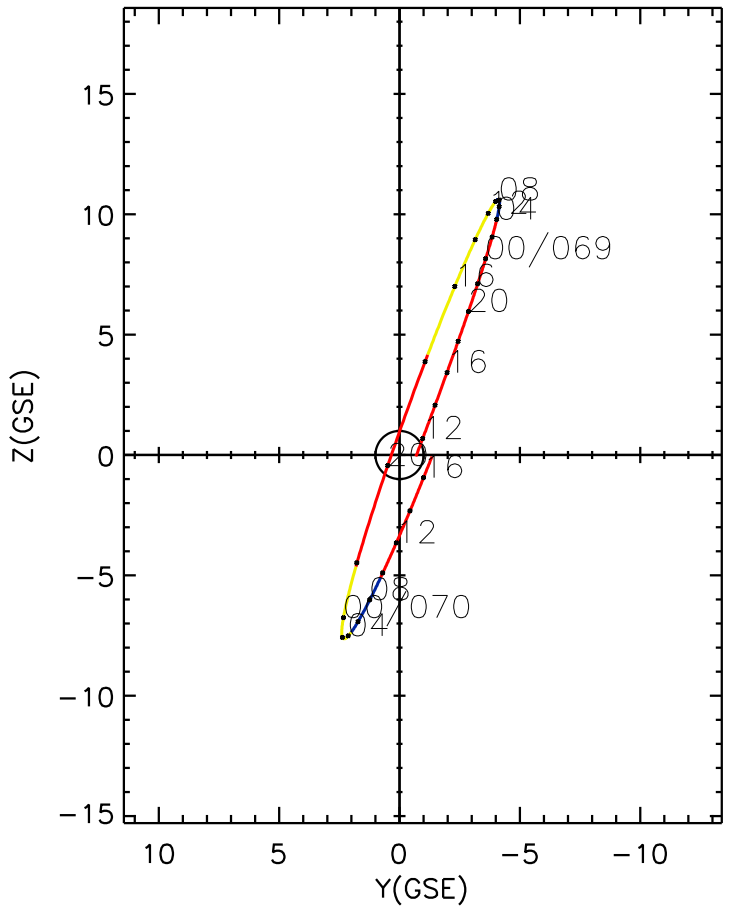
CLUSTER 2 orbit 2020 068 (03/08) 10:56 UT to 2020 070 (03/10) 17:16 UT
