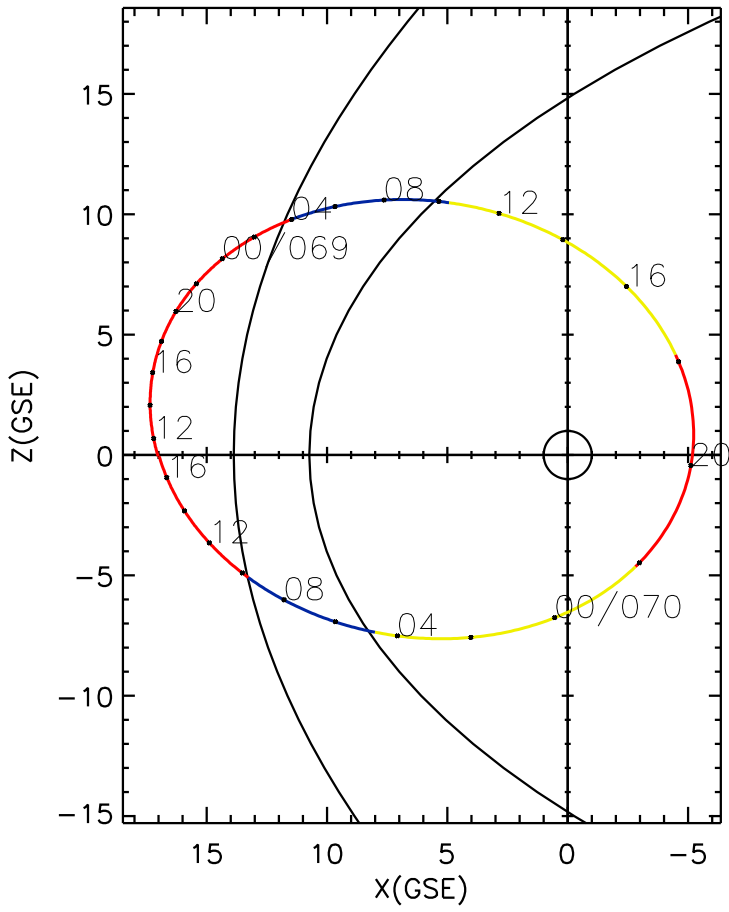
CLUSTER 2 orbit 2020 068 (03/08) 10:56 UT to 2020 070 (03/10) 17:16 UT
