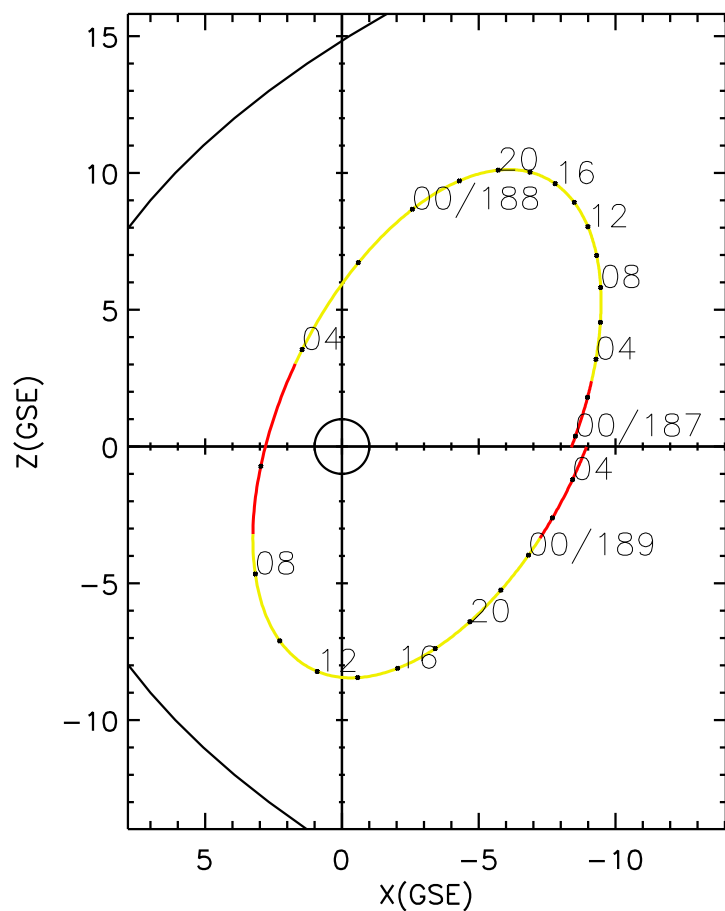
CLUSTER 2 orbit 2019 186 (07/05) 23:26 UT to 2019 189 (07/08) 05:41 UT
