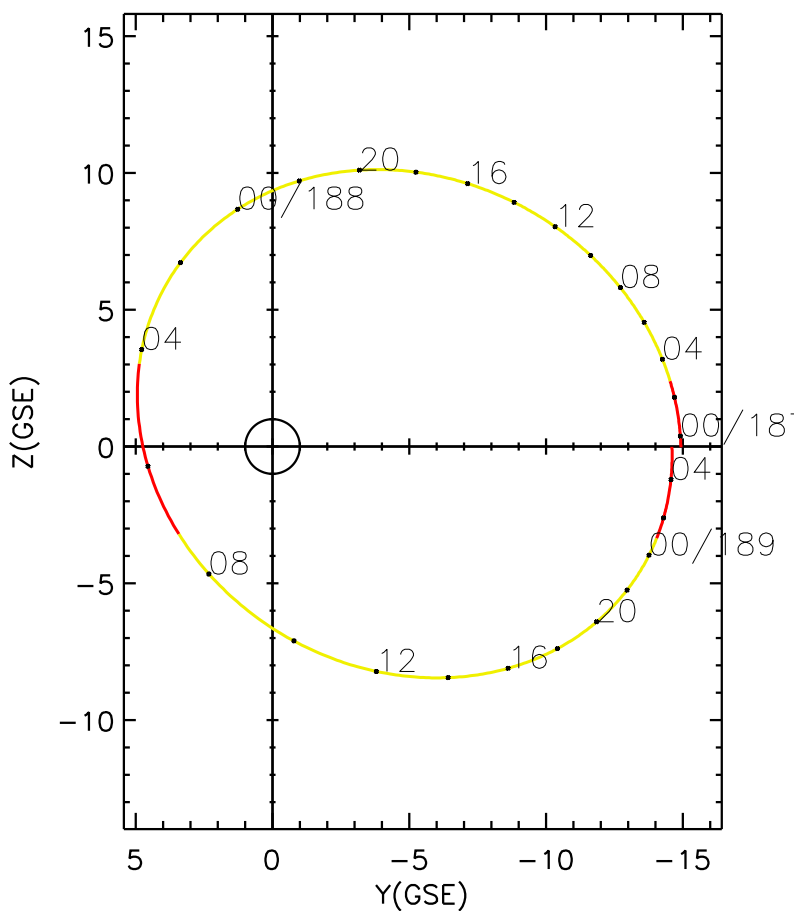
CLUSTER 2 orbit 2019 186 (07/05) 23:26 UT to 2019 189 (07/08) 05:41 UT
