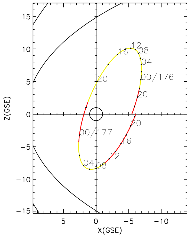
CLUSTER 2 orbit 2019 175 (06/24) 16:16 UT to 2019 177 (06/26) 22:31 UT
