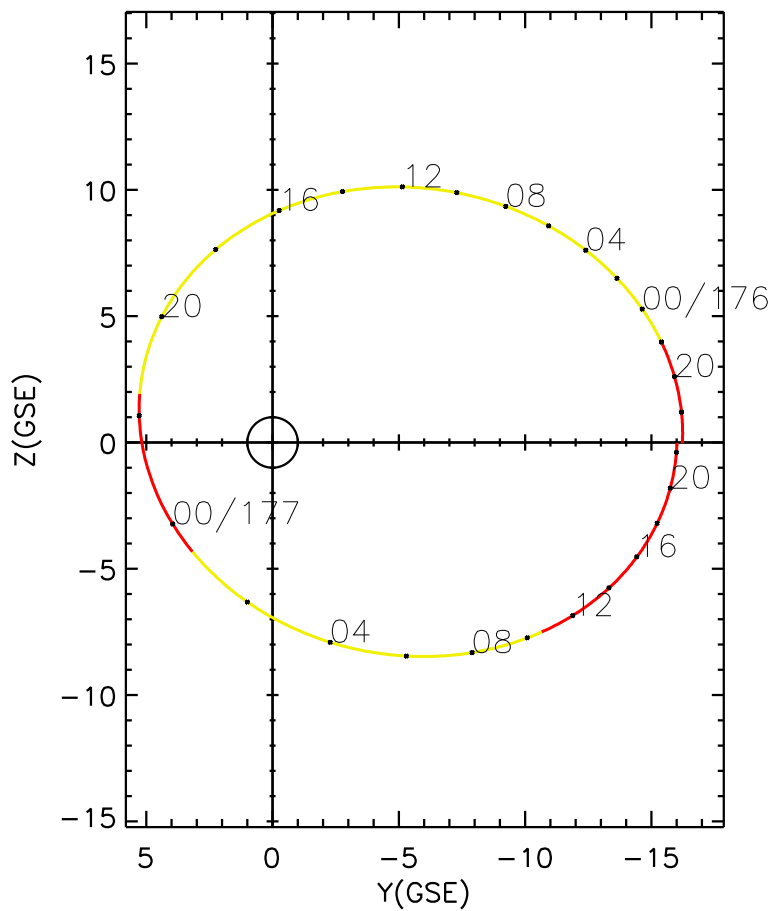
CLUSTER 2 orbit 2019 175 (06/24) 16:16 UT to 2019 177 (06/26) 22:31 UT
