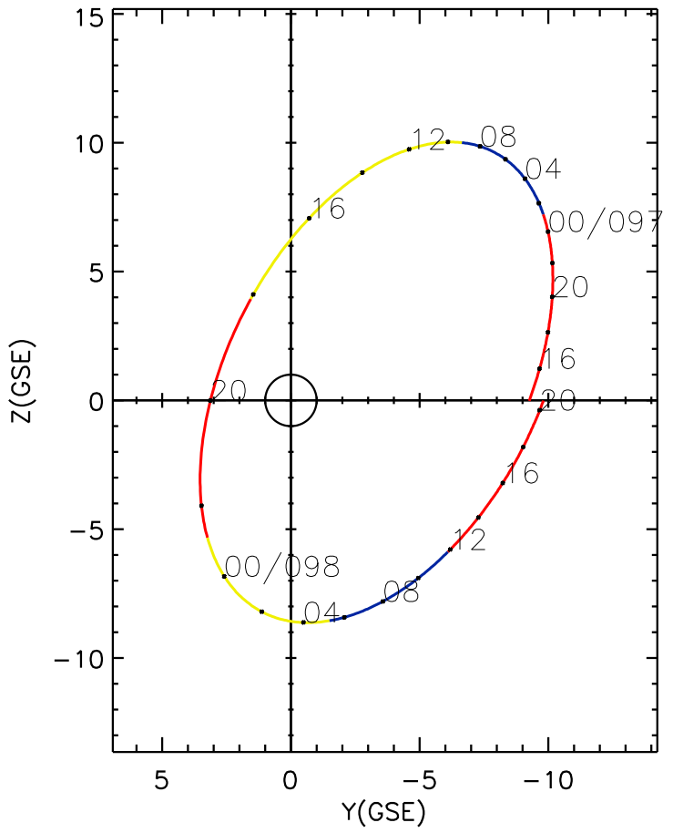
CLUSTER 2 orbit 2019 096 (04/06) 14:16 UT to 2019 098 (04/08) 20:31 UT
