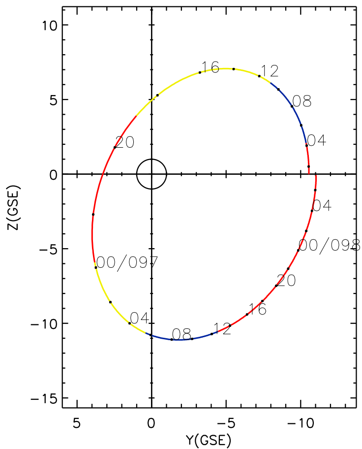
CLUSTER 2 orbit 2016 096 (04/05) 01:16 UT to 2016 098 (04/07) 07:26 UT
