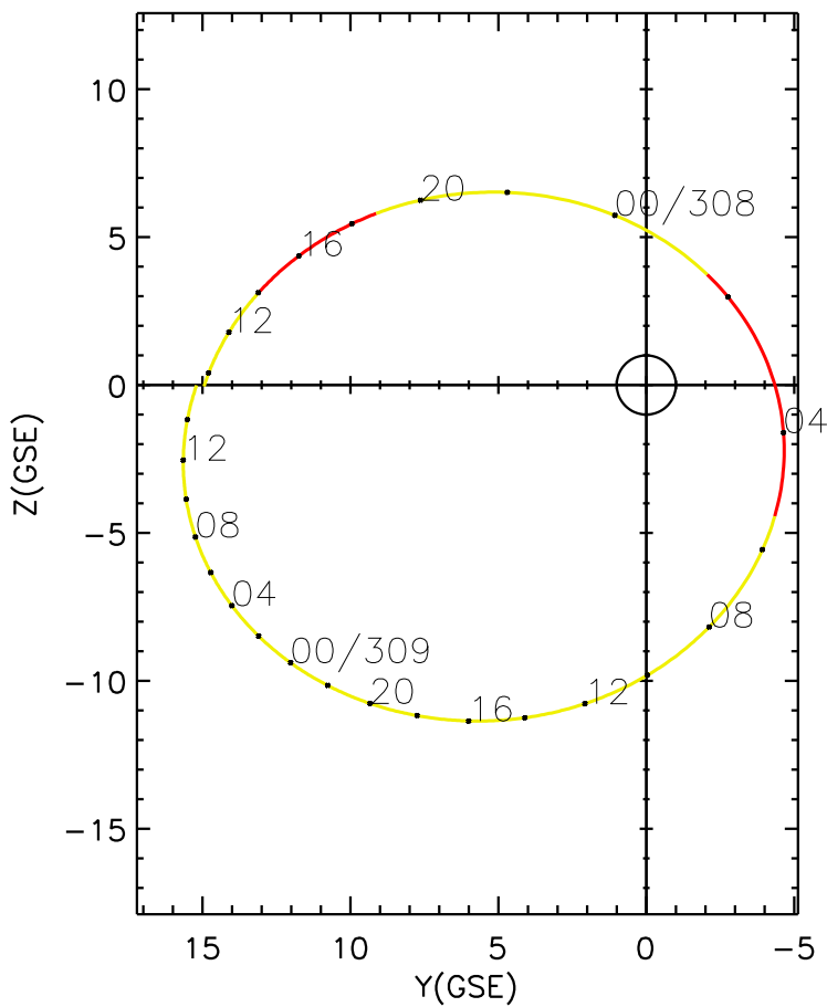
CLUSTER 2 orbit 2015 307 (11/03) 09:21 UT to 2015 309 (11/05) 15:41 UT
