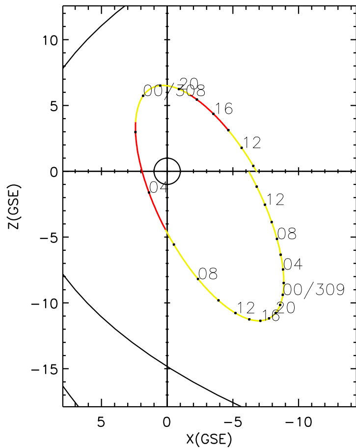
CLUSTER 2 orbit 2015 307 (11/03) 09:21 UT to 2015 309 (11/05) 15:41 UT
