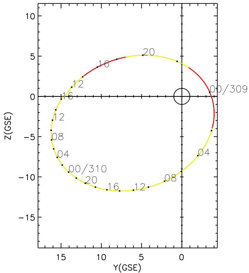
CLUSTER 2 orbit 2014 308 (11/04) 10:11 UT to 2014 310 (11/06) 16:31 UT
