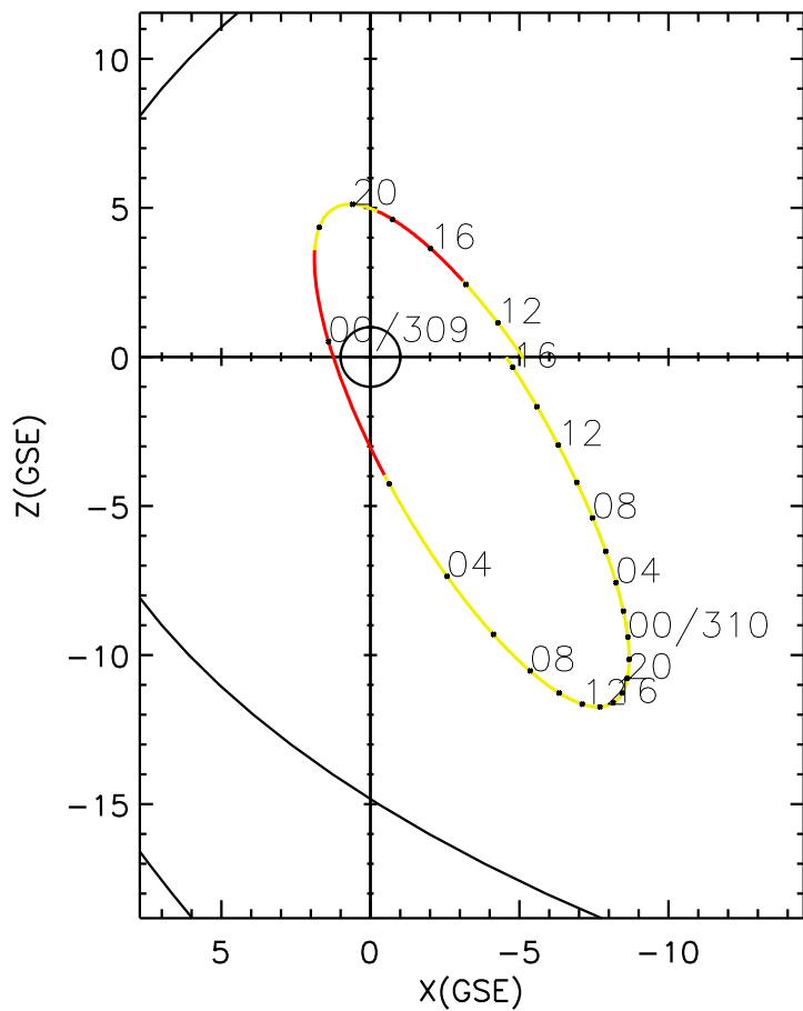
CLUSTER 2 orbit 2014 308 (11/04) 10:11 UT to 2014 310 (11/06) 16:31 UT
