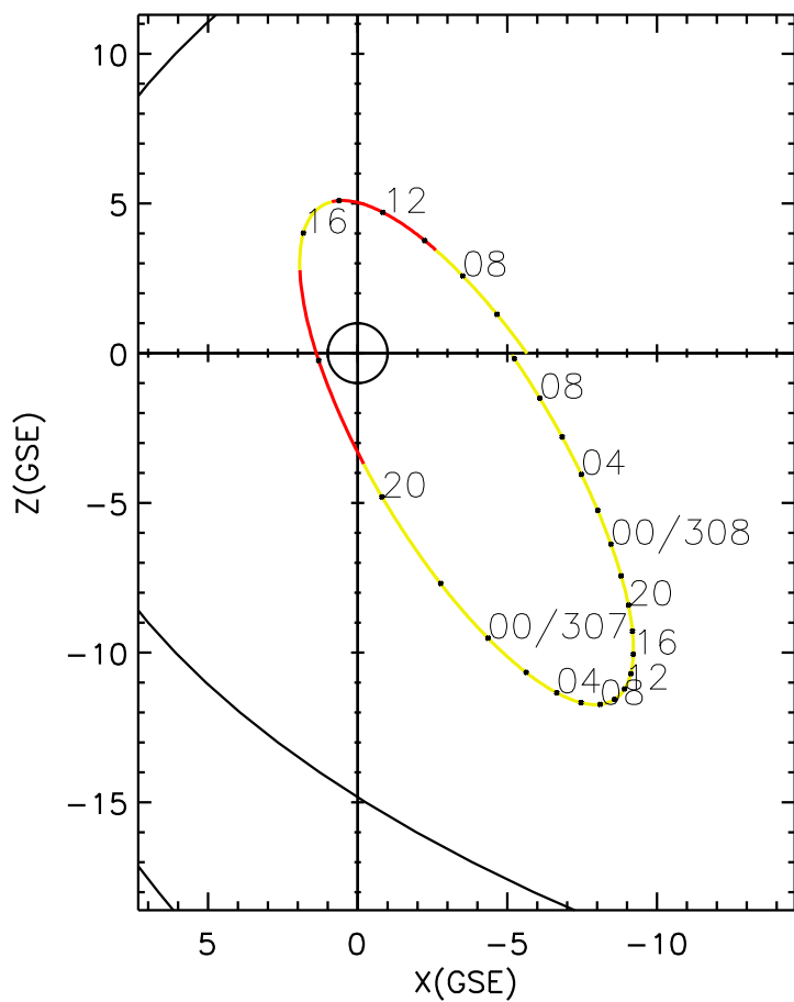
CLUSTER 2 orbit 2014 306 (11/02) 04:01 UT to 2014 308 (11/04) 10:11 UT
