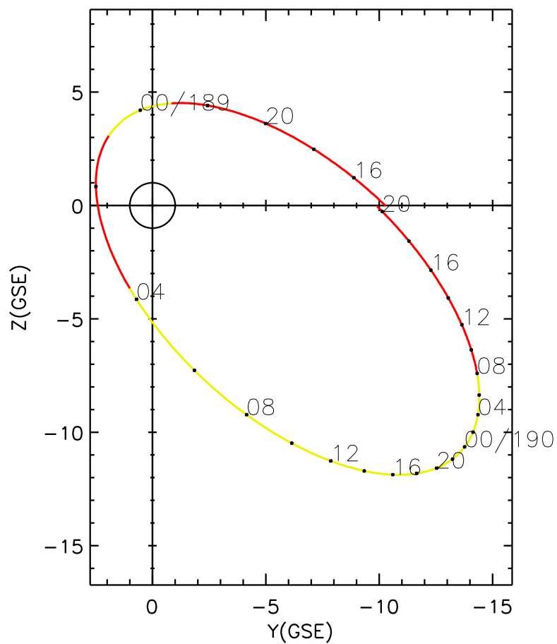
CLUSTER 2 orbit 2014 188 (07/07) 14:06 UT to 2014 190 (07/09) 20:21 UT
