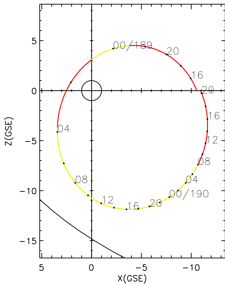
CLUSTER 2 orbit 2014 188 (07/07) 14:06 UT to 2014 190 (07/09) 20:21 UT
