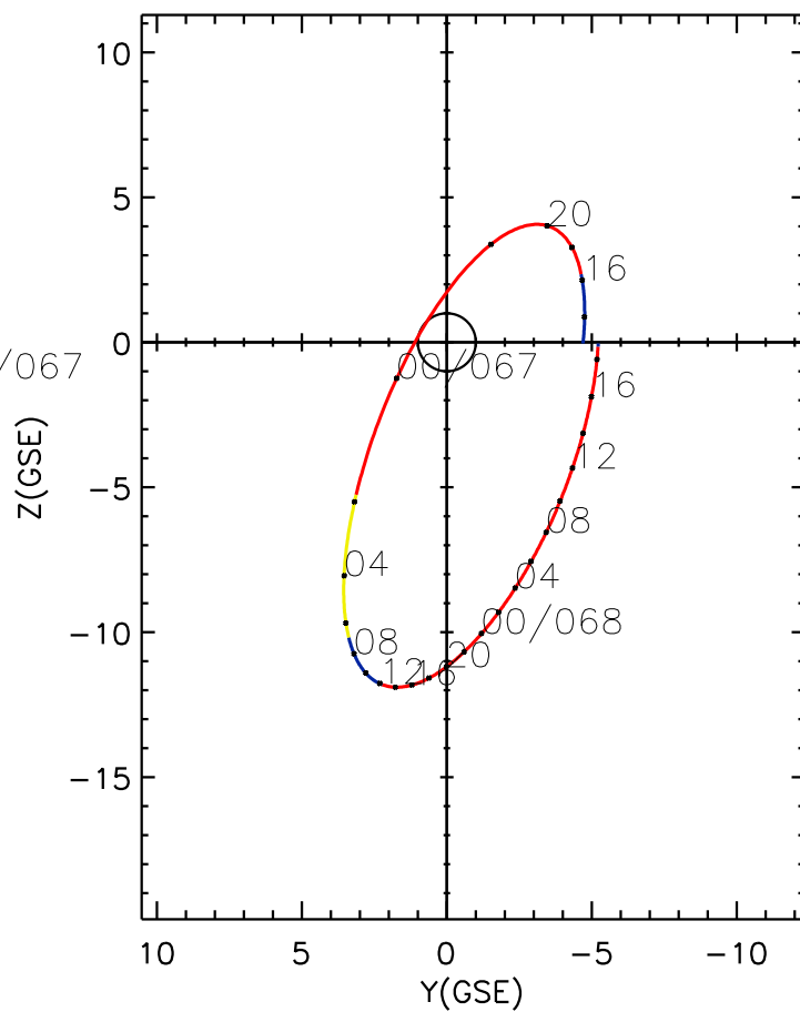
CLUSTER 2 orbit 2014 066 (03/07) 12:36 UT to 2014 068 (03/09) 18:51 UT
