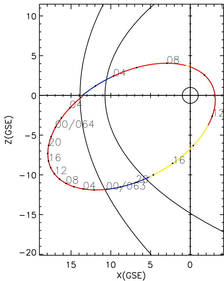
CLUSTER 2 orbit 2014 062 (03/03) 00:06 UT to 2014 064 (03/05) 06:21 UT
