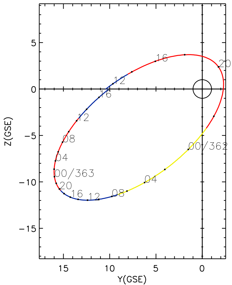
CLUSTER 2 orbit 2013 361 (12/27) 11:06 UT to 2013 363 (12/29) 17:21 UT
