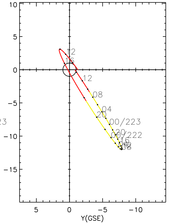
CLUSTER 2 orbit 2013 221 (08/09) 08:16 UT to 2013 223 (08/11) 14:31 UT
