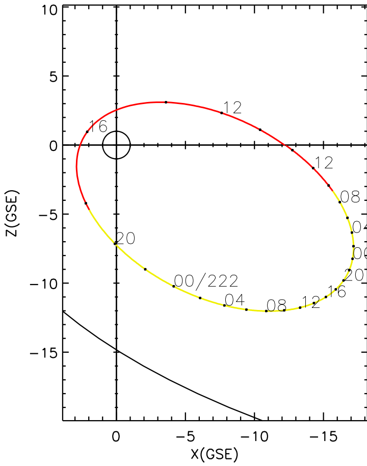
CLUSTER 2 orbit 2013 221 (08/09) 08:16 UT to 2013 223 (08/11) 14:31 UT
