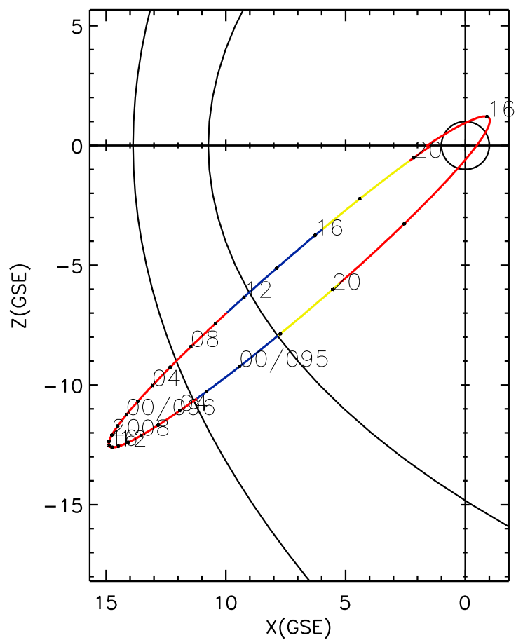
CLUSTER 2 orbit 2012 094 (04/03) 14:16 UT to 2012 096 (04/05) 20:31 UT
