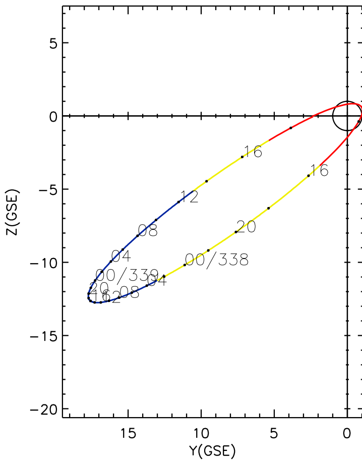
CLUSTER 2 orbit 2011 337 (12/03) 12:26 UT to 2011 339 (12/05) 18:41 UT
