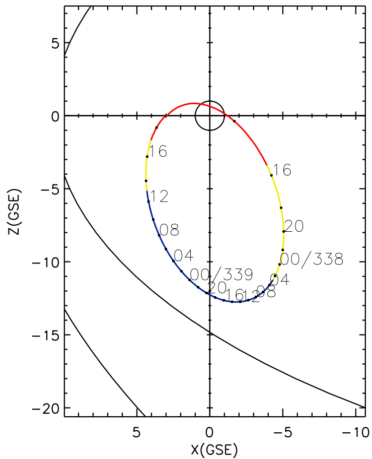
CLUSTER 2 orbit 2011 337 (12/03) 12:26 UT to 2011 339 (12/05) 18:41 UT
