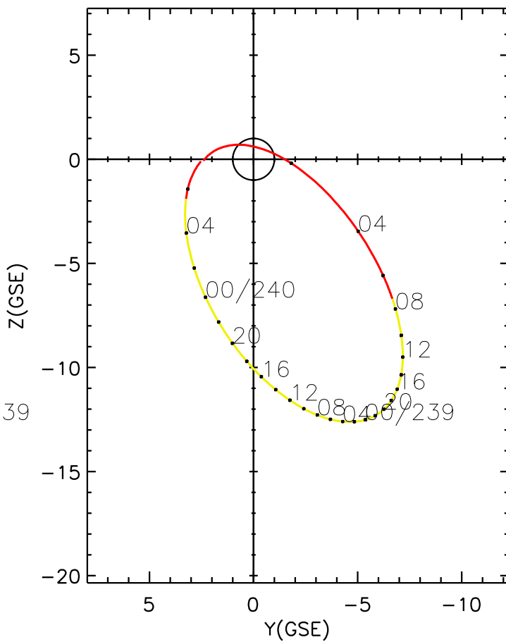
CLUSTER 2 orbit 2011 238 (08/26) 00:46 UT to 2011 240 (08/28) 07:01 UT
