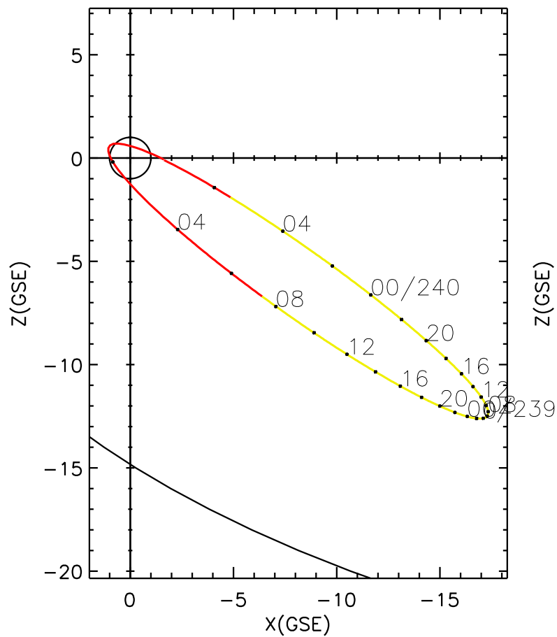
CLUSTER 2 orbit 2011 238 (08/26) 00:46 UT to 2011 240 (08/28) 07:01 UT
