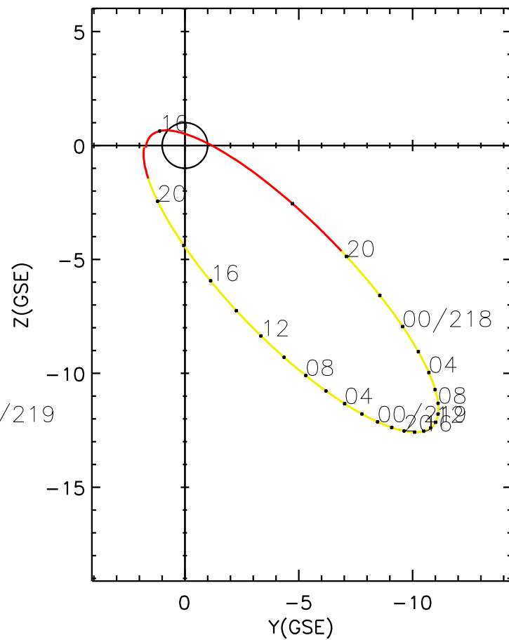
CLUSTER 2 orbit 2011 217 (08/05) 15:26 UT to 2011 219 (08/07) 21:51 UT
