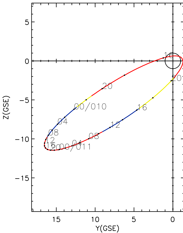
CLUSTER 2 orbit 2011 009 (01/09) 15:11 UT to 2011 011 (01/11) 21:26 UT
