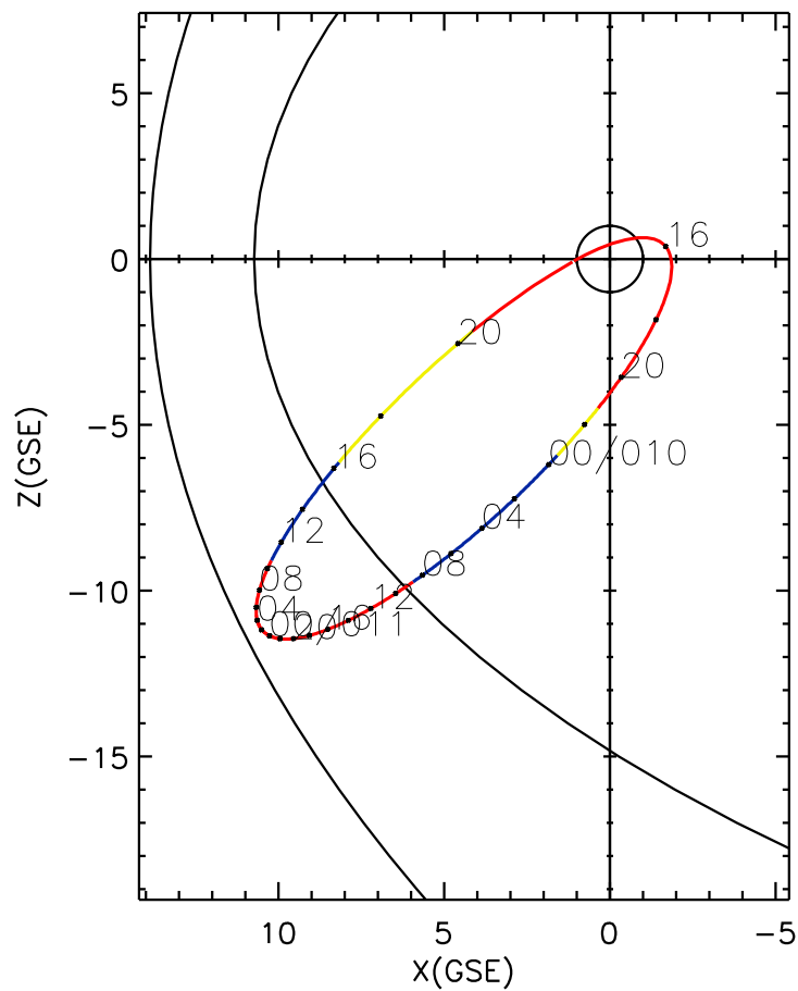
CLUSTER 2 orbit 2011 009 (01/09) 15:11 UT to 2011 011 (01/11) 21:26 UT
