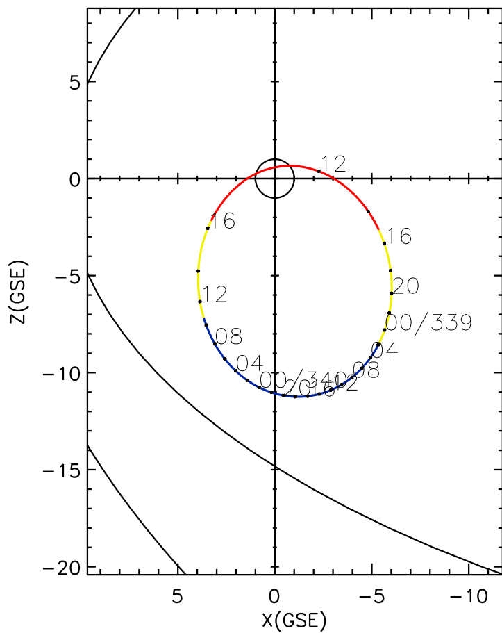
CLUSTER 2 orbit 2010 338 (12/04) 11:06 UT to 2010 340 (12/06) 17:21 UT
