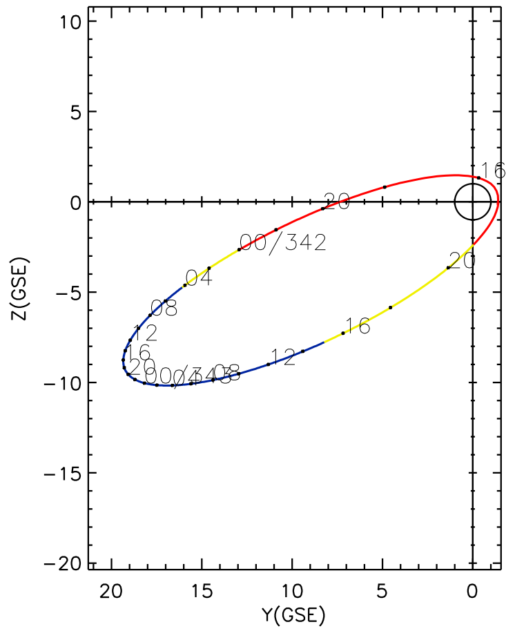
CLUSTER 2 orbit 2009 341 (12/07) 15:21 UT to 2009 343 (12/09) 21:41 UT
