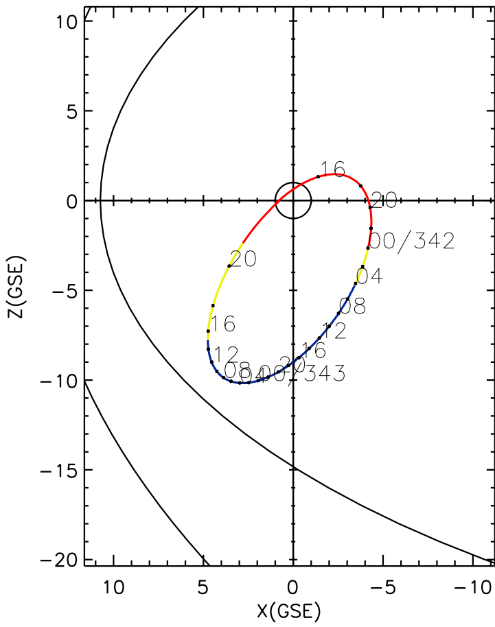
CLUSTER 2 orbit 2009 341 (12/07) 15:21 UT to 2009 343 (12/09) 21:41 UT
