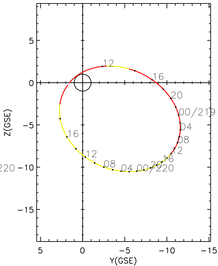
CLUSTER 2 orbit 2009 218 (08/06) 10:51 UT to 2009 220 (08/08) 19:56 UT
