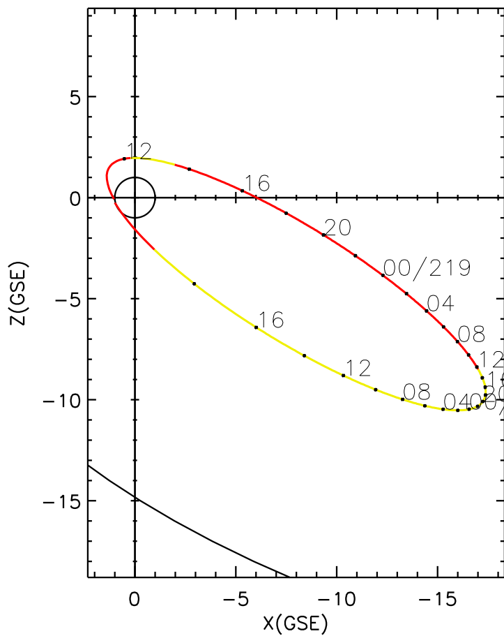
CLUSTER 2 orbit 2009 218 (08/06) 10:51 UT to 2009 220 (08/08) 19:56 UT
