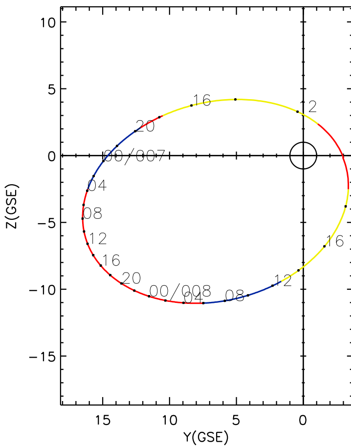
CLUSTER 2 orbit 2008 006 (01/06) 10:26 UT to 2008 008 (01/08) 19:31 UT
