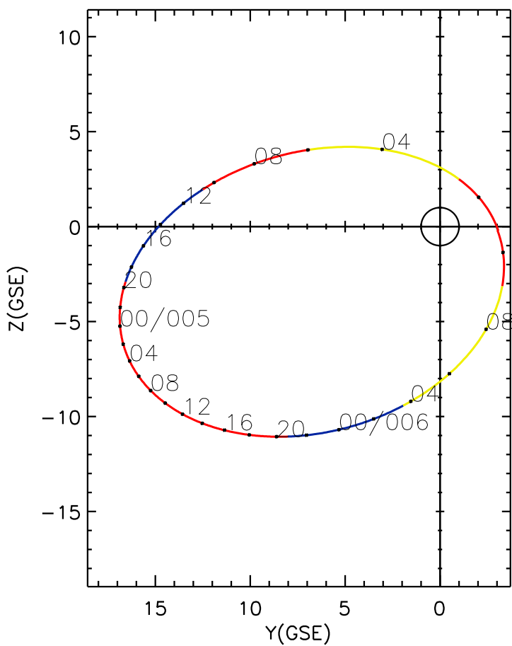
CLUSTER 2 orbit 2008 004 (01/04) 01:21 UT to 2008 006 (01/06) 10:26 UT
