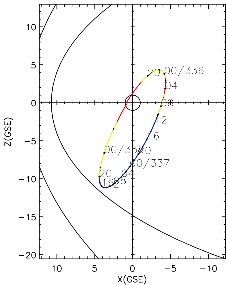
CLUSTER 2 orbit 2007 335 (12/01) 18:15 UT to 2007 338 (12/04) 03:20 UT
