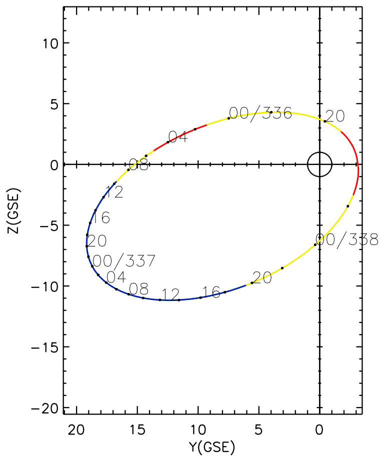
CLUSTER 2 orbit 2007 335 (12/01) 18:15 UT to 2007 338 (12/04) 03:20 UT
