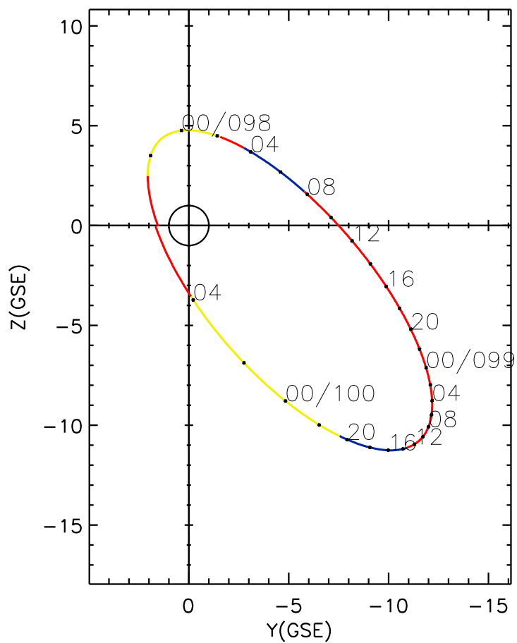
CLUSTER 2 orbit 2007 097 (04/07) 20:25 UT to 2007 100 (04/10) 05:30 UT
