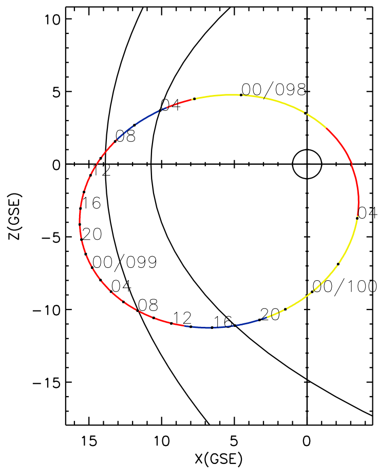
CLUSTER 2 orbit 2007 097 (04/07) 20:25 UT to 2007 100 (04/10) 05:30 UT
