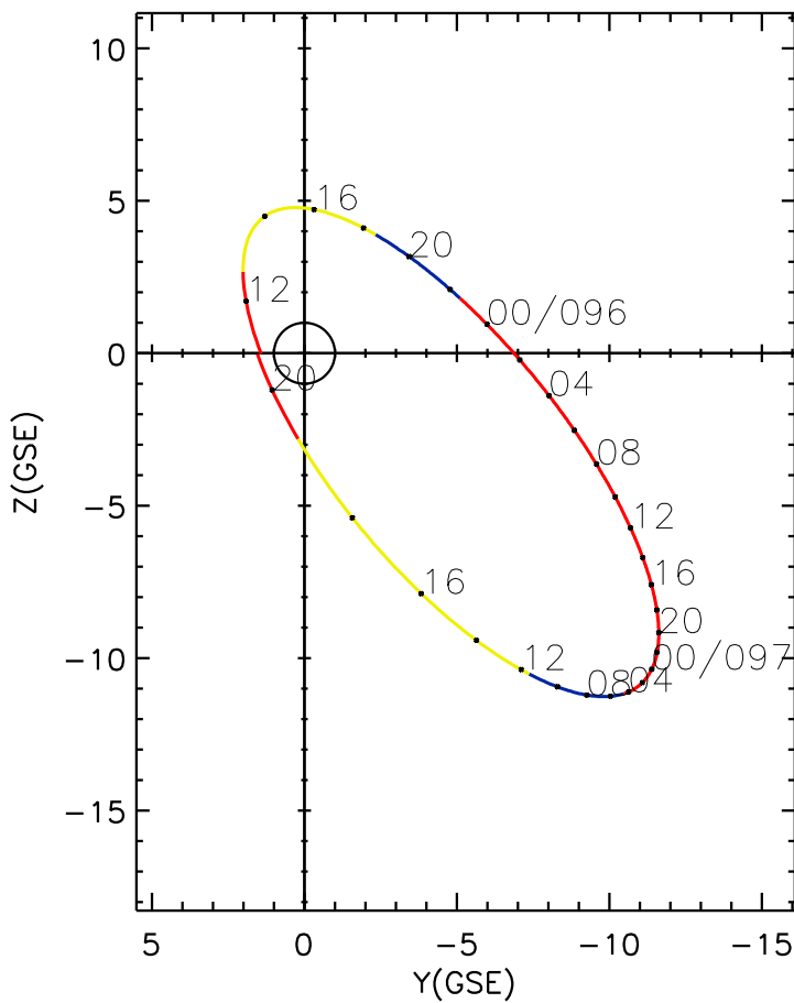
CLUSTER 2 orbit 2007 095 (04/05) 11:21 UT to 2007 097 (04/07) 20:26 UT
