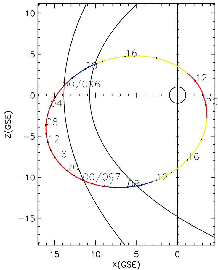
CLUSTER 2 orbit 2007 095 (04/05) 11:21 UT to 2007 097 (04/07) 20:26 UT
