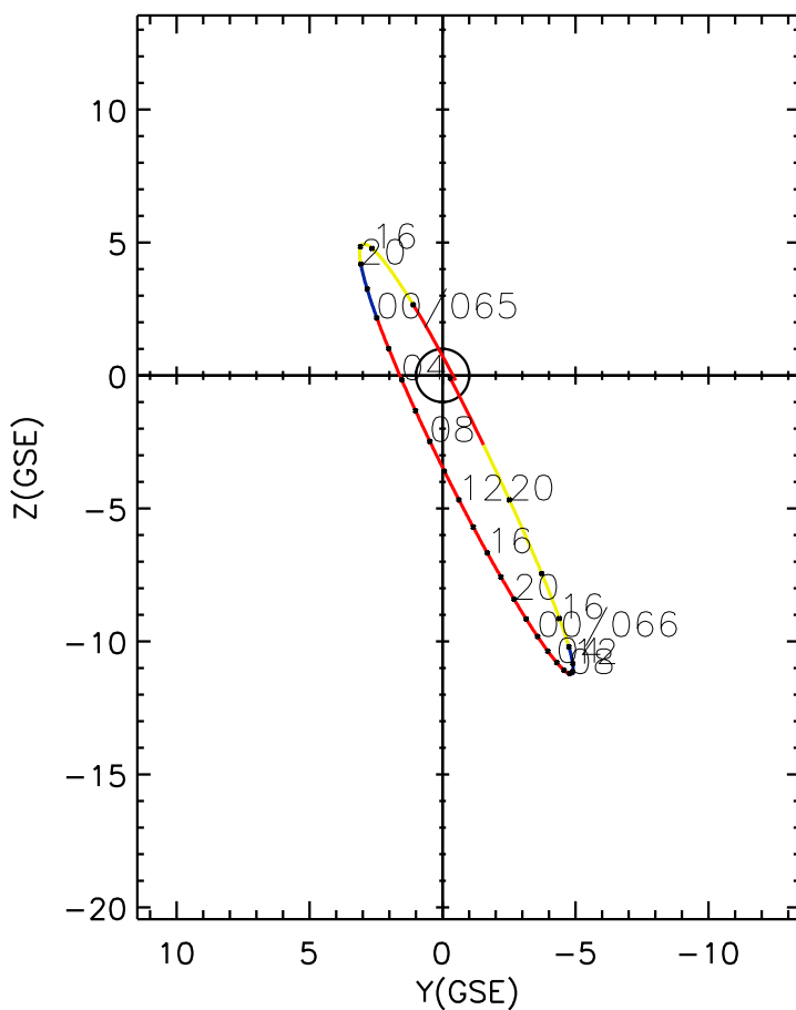
CLUSTER 2 orbit 2007 064 (03/05) 12:51 UT to 2007 066 (03/07) 22:01 UT
