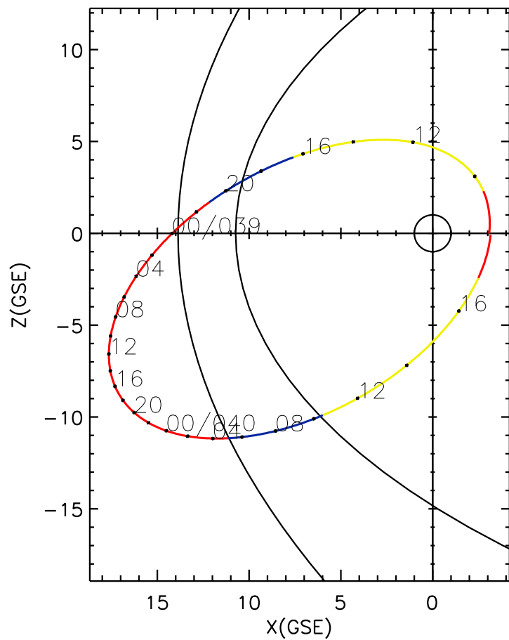
CLUSTER 2 orbit 2007 038 (02/07) 08:41 UT to 2007 040 (02/09) 17:46 UT
