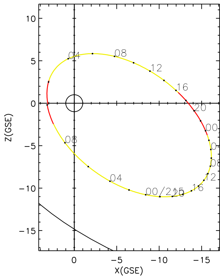
CLUSTER 2 orbit 2006 213 (08/01) 00:55 UT to 2006 215 (08/03) 10:00 UT
