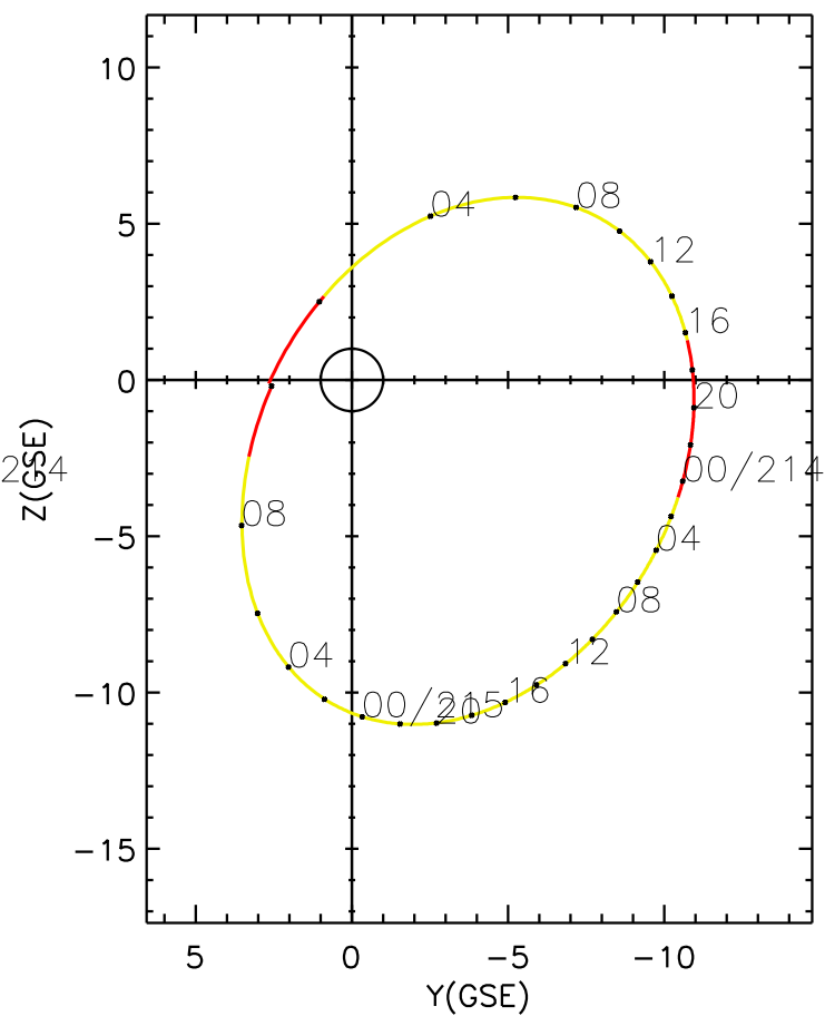
CLUSTER 2 orbit 2006 213 (08/01) 00:55 UT to 2006 215 (08/03) 10:00 UT
