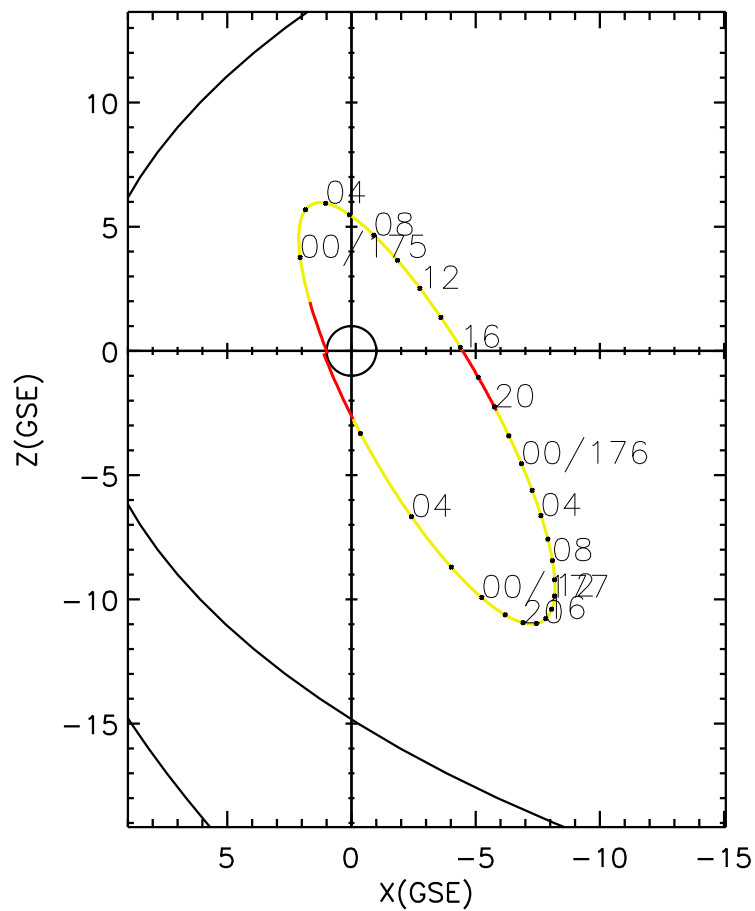
CLUSTER 2 orbit 2006 174 (06/23) 22:16 UT to 2006 177 (06/26) 07:21 UT
