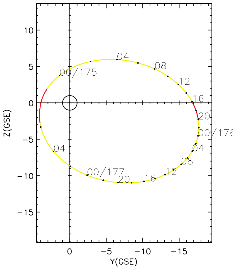
CLUSTER 2 orbit 2006 174 (06/23) 22:16 UT to 2006 177 (06/26) 07:21 UT
