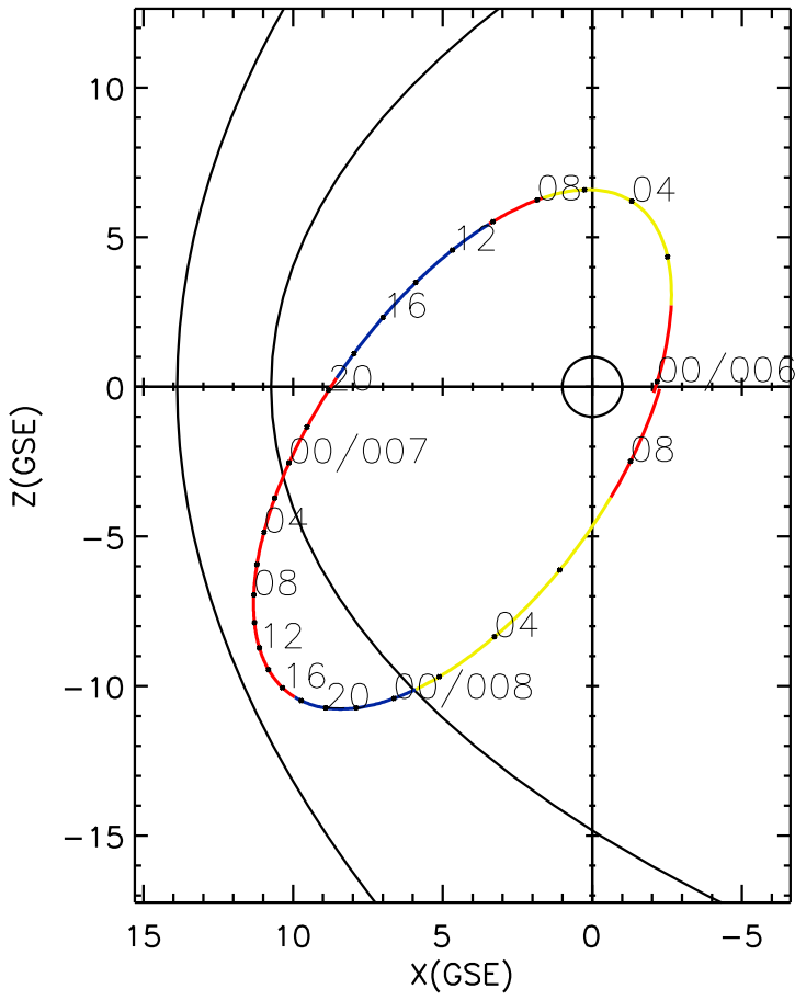
CLUSTER 2 orbit 2006 005 (01/05) 23:51 UT to 2006 008 (01/08) 09:01 UT
