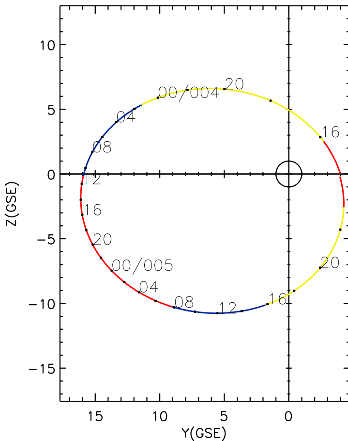
CLUSTER 2 orbit 2006 003 (01/03) 14:46 UT to 2006 005 (01/05) 23:51 UT
