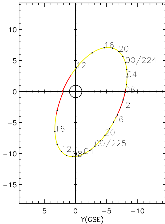
CLUSTER 2 orbit 2005 223 (08/11) 10:11 UT to 2005 225 (08/13) 19:16 UT
