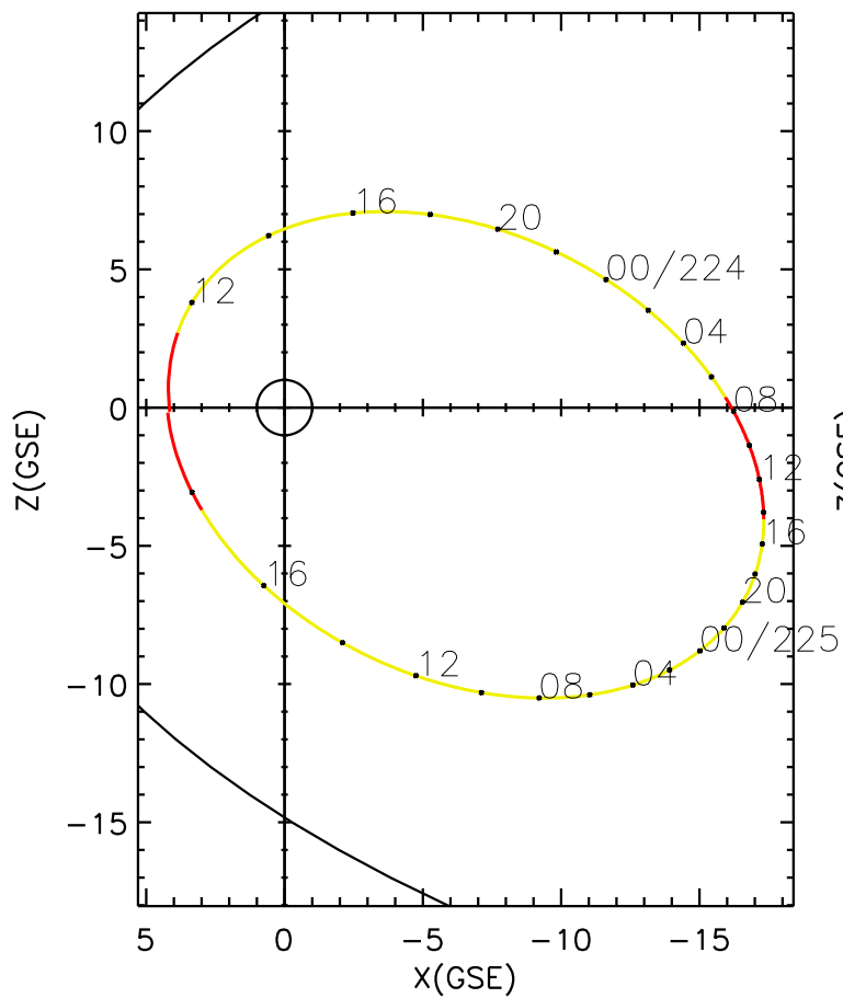
CLUSTER 2 orbit 2005 223 (08/11) 10:11 UT to 2005 225 (08/13) 19:16 UT
