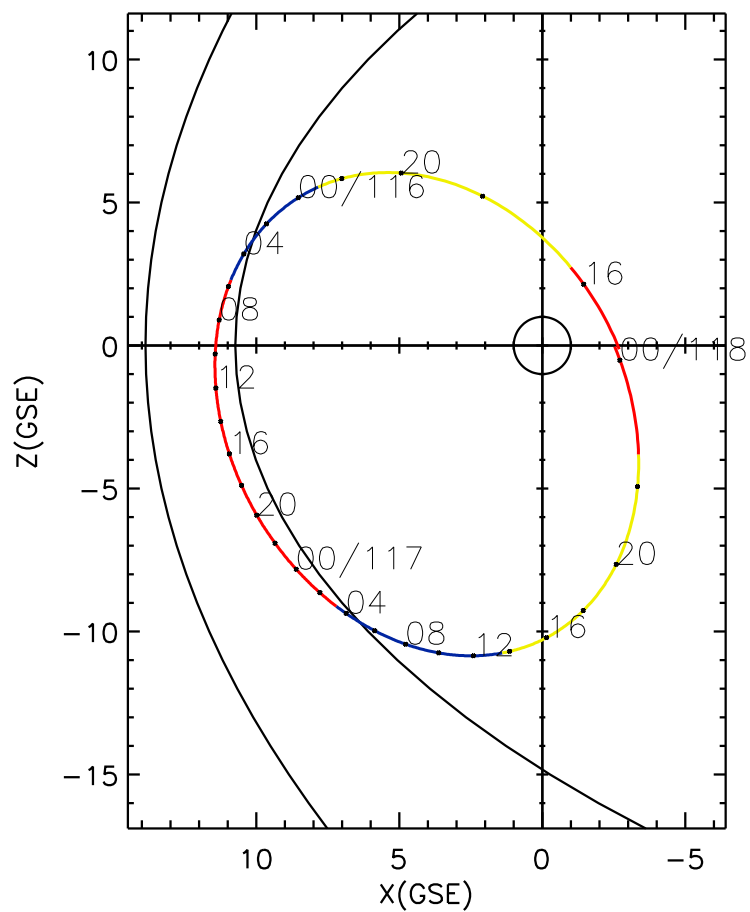
CLUSTER 2 orbit 2005 115 (04/25) 15:05 UT to 2005 118 (04/28) 00:11 UT
