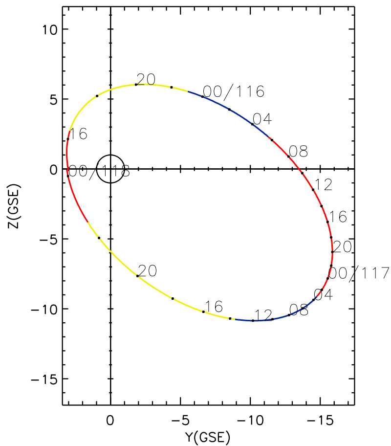
CLUSTER 2 orbit 2005 115 (04/25) 15:05 UT to 2005 118 (04/28) 00:11 UT
