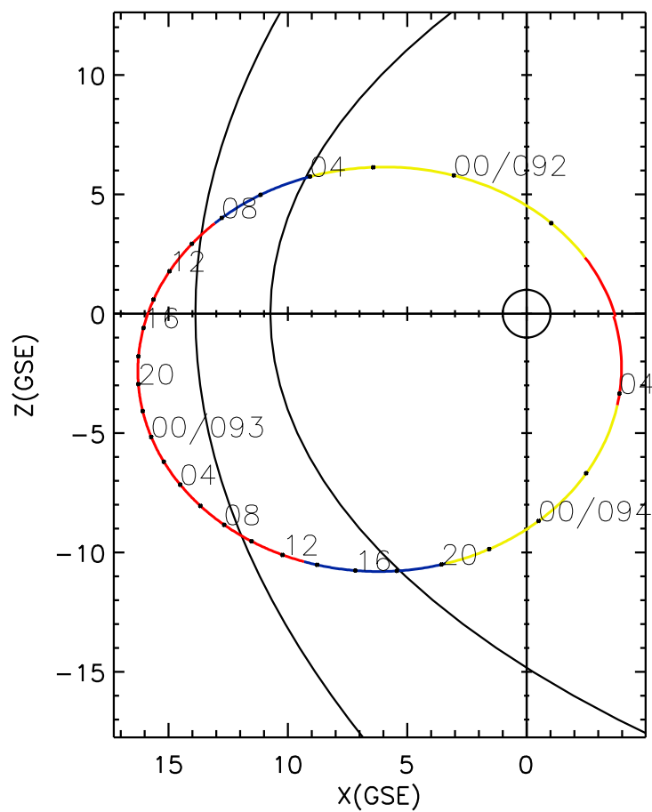
CLUSTER 2 orbit 2005 091 (04/01) 20:16 UT to 2005 094 (04/04) 05:21 UT
