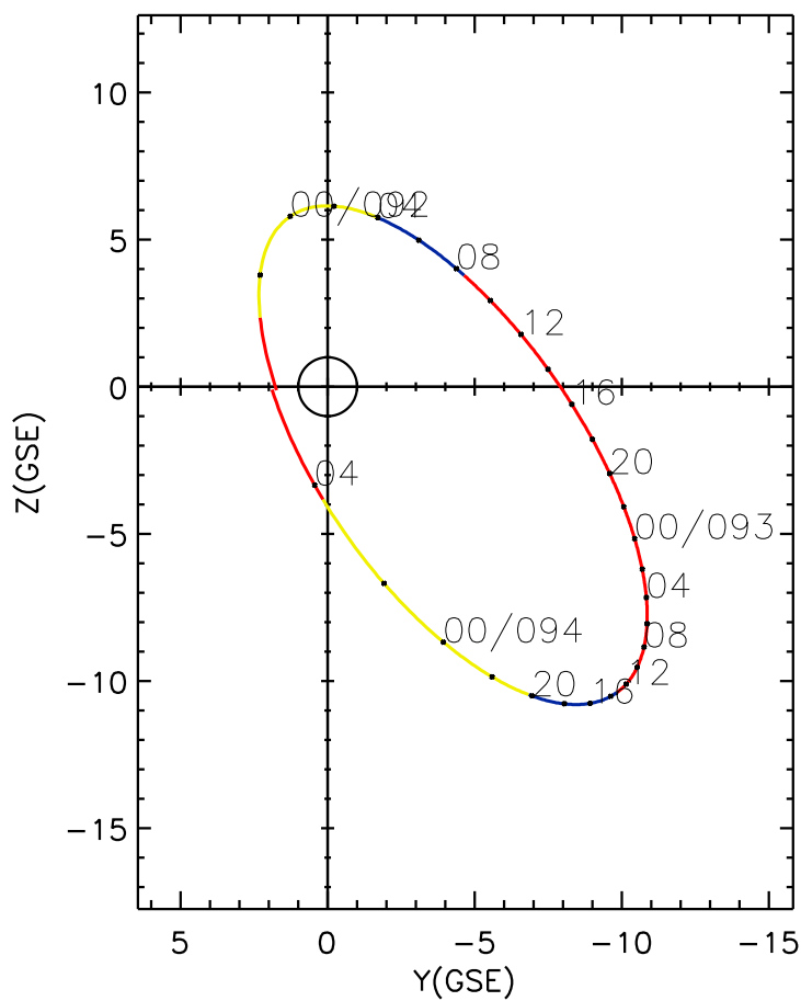
CLUSTER 2 orbit 2005 091 (04/01) 20:16 UT to 2005 094 (04/04) 05:21 UT
